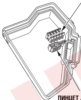
ПИНЦЕТ ДЛЯ СЪЕМА ПРЕДОХРАНИТЕЛЕЙ
