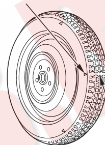
ИНДИКАТОР ПРЕДЕЛЬНОГО ИЗНОСА ПРОТЕКТОРА
