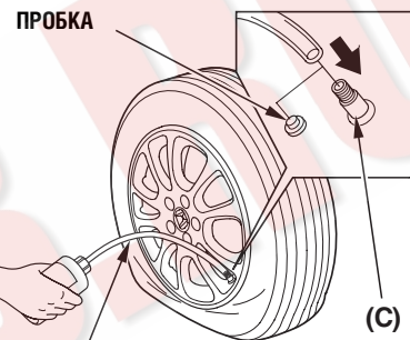
ЗАПРАВОЧНЫЙ ШЛАНГ
